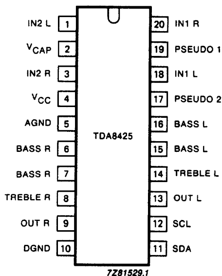
Fig.2 Pinning diagram.
